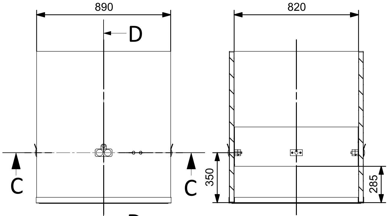
SECTION D-D
