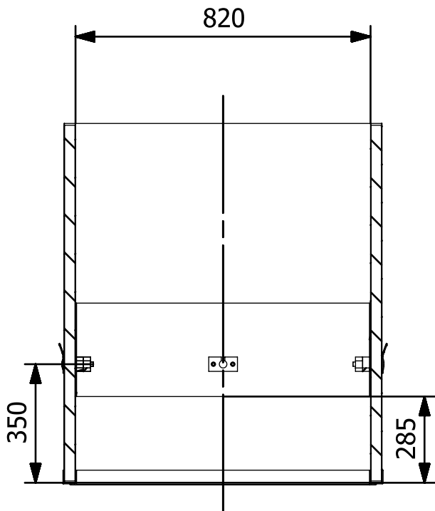
SECTION D-D
